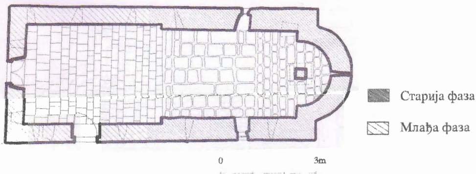
Основа цркве са изгледом пода
