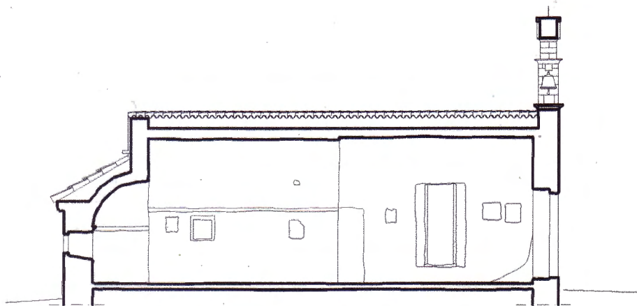
Подужни пресјек са погледом на јужну страну
